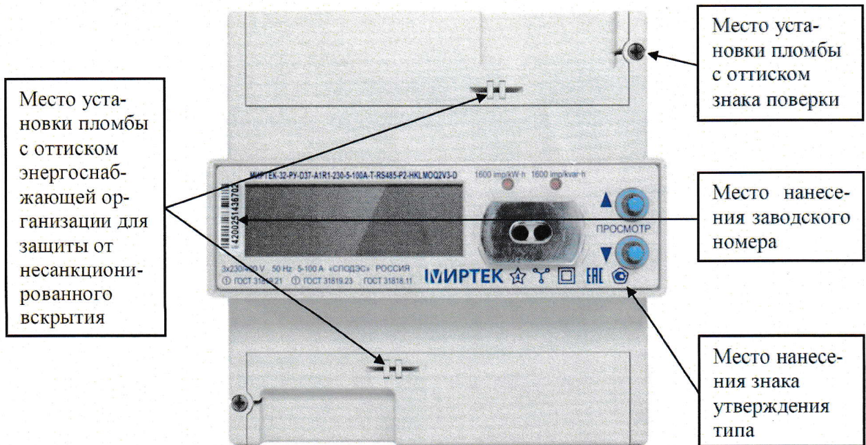
Рисунок 8 – Общий вид счетчика в корпусе типа D37
