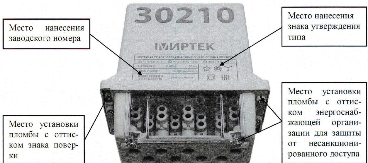
Рисунок 9 – Общий вид счетчика в корпусе типа SP31
