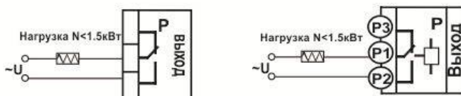
Подключение нагрузки менее 1,5 кВт
