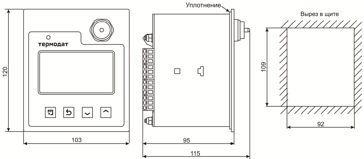
Рисунок 14 – Габаритные размеры прибора Термодат-16E6/...../IP67пп или Термодат-16E6-A7
