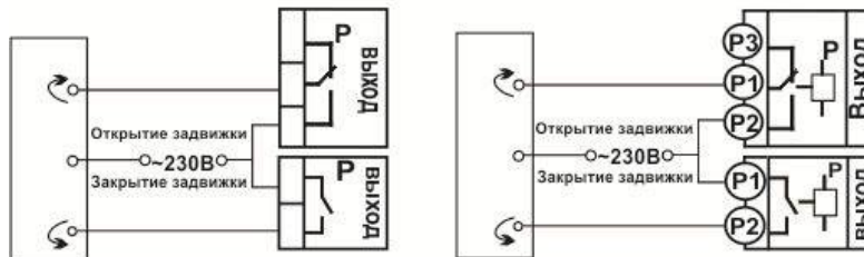
Подключение электрозадвижки
