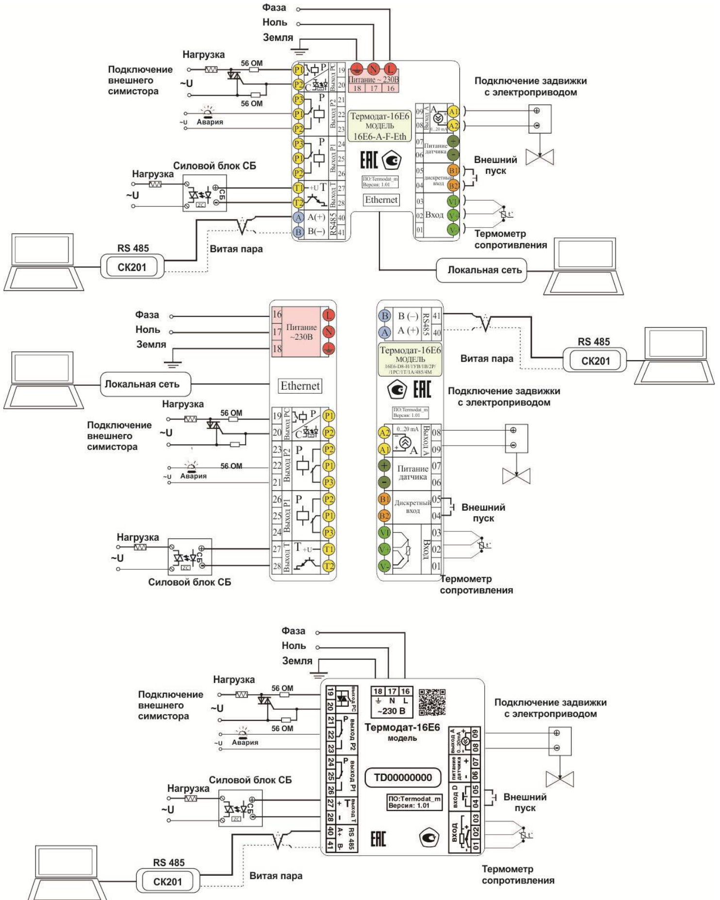
Рисунок 12 – Схема подключения прибора
