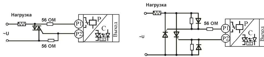
Подключение внешнего симистора
